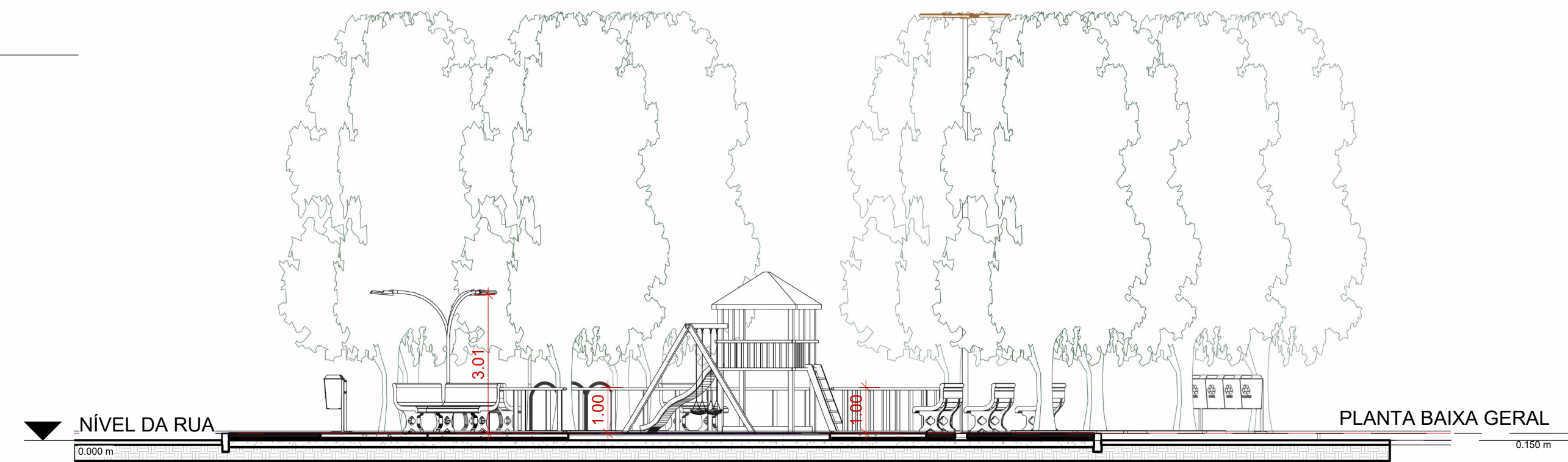
6 Corte B 1 : 100
