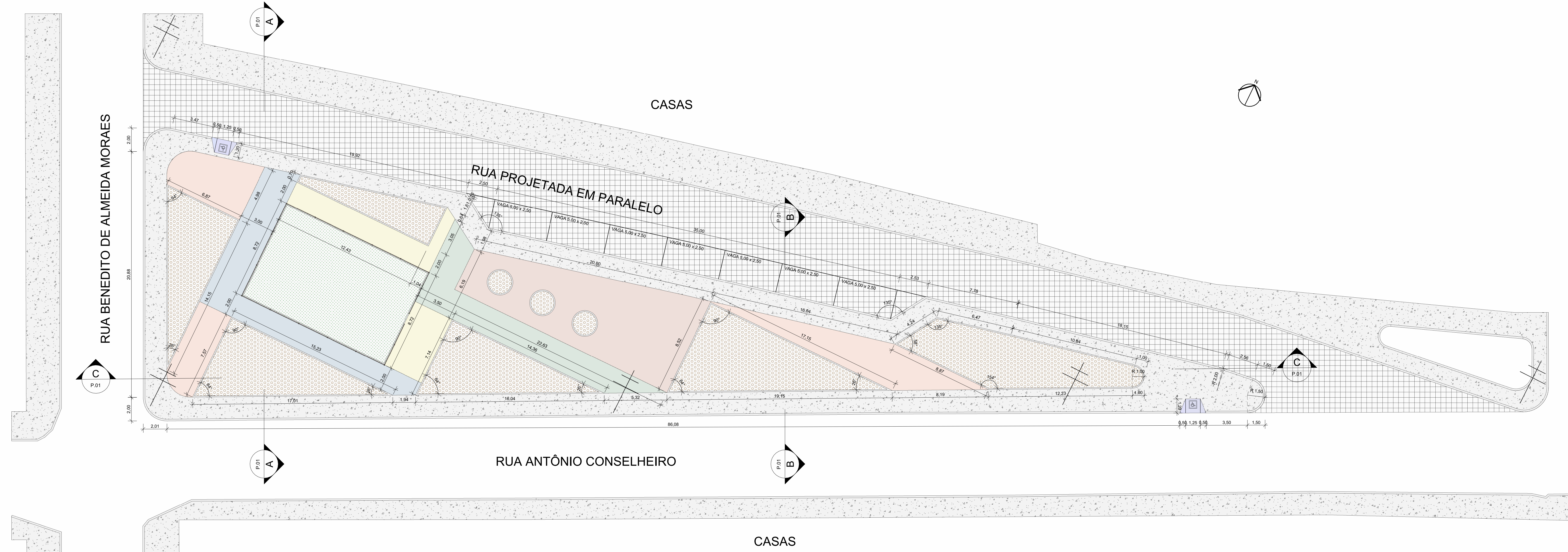
1 PLANTA BAIXA COTADA 1 : 150
