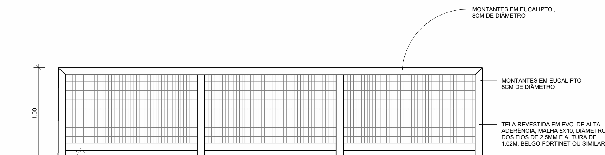
6 DETALHAMENTO CERCA PARQUINHO 1 : 25
