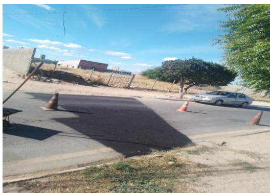
AV JOÃO PAULO II - TAPA BURACO CBUQ
