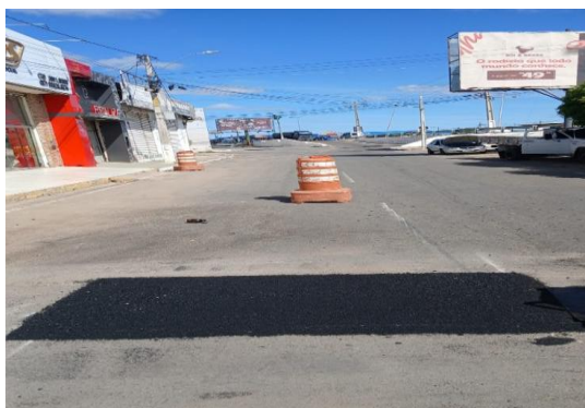
AV SANTOS DUMONT - APLICAÇÃO DE CBUQ
