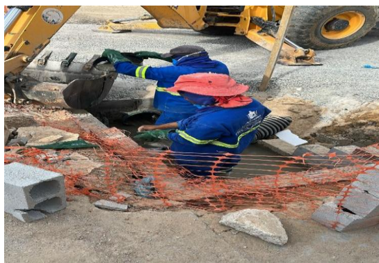
AV PROPRIÁ - APLICAÇÃO DE BGS
