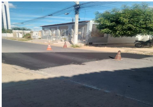
RUA SÃO JOÃO - TAPA BURACO CBUQ
