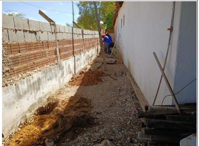
- Escavação para fixação de pilaretes para amarração do muro.
