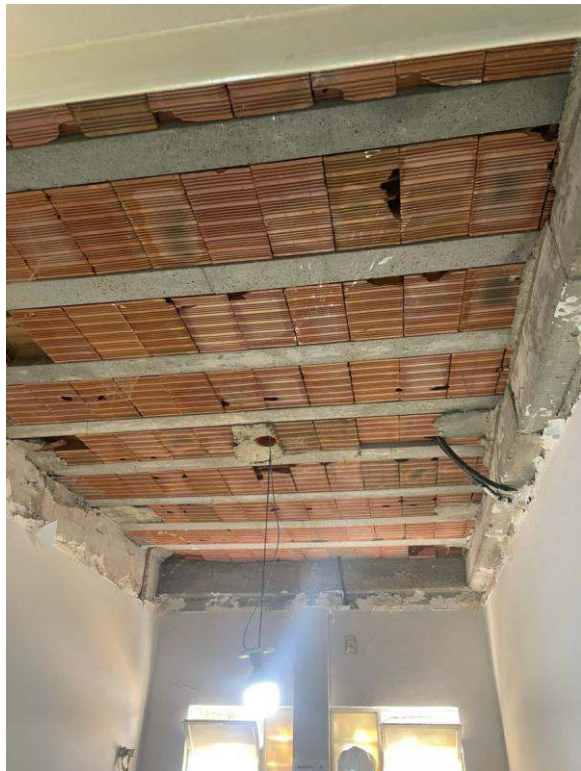
- Demolição do forro de gesso da copa
