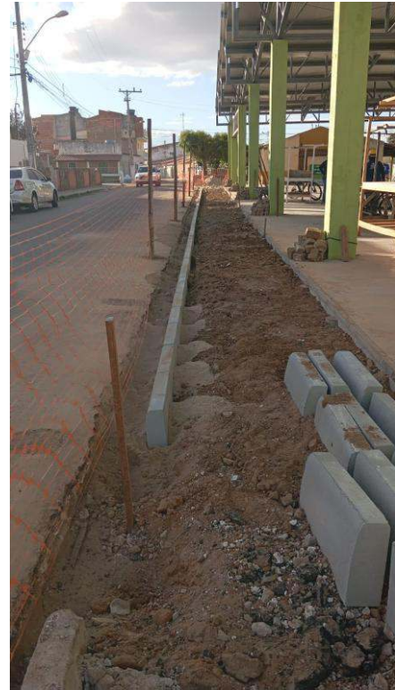
- Assentamento de meio fio
