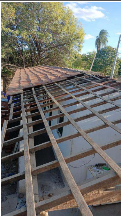
- Remoção de telhado para reparos
