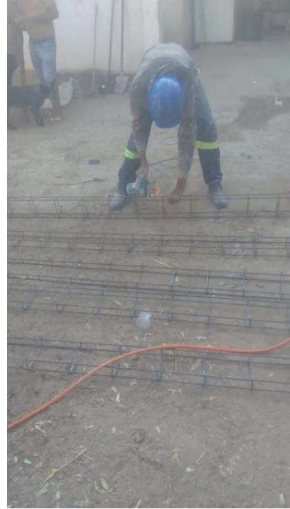
- Preparação de ferragem do muro
