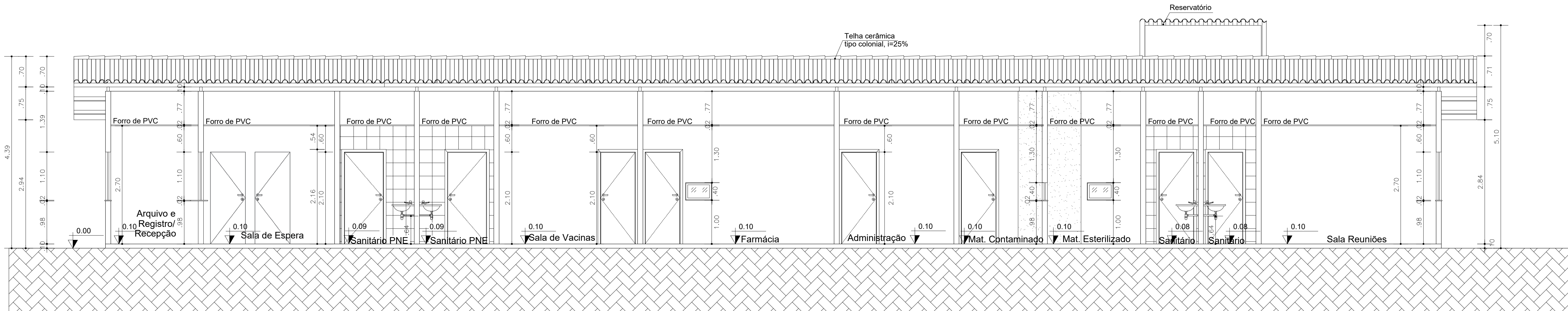
CORTE AA ESCALA: 1/75
