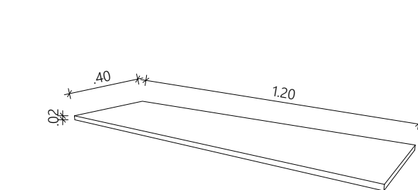
VISTA ISOMÉTRICA SEM ESCALA
