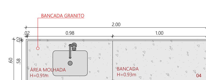
VISTA SUPERIOR SEM ESCALA
