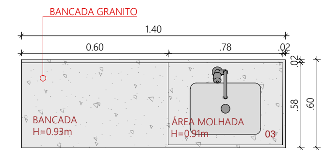
VISTA SUPERIOR SEM ESCALA
