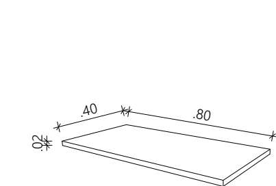
VISTA ISOMÉTRICA SEM ESCALA
