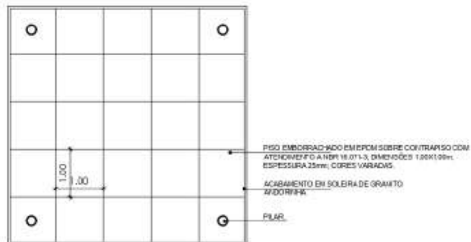
PLANTA BAIXA - EMBORRACHADO
