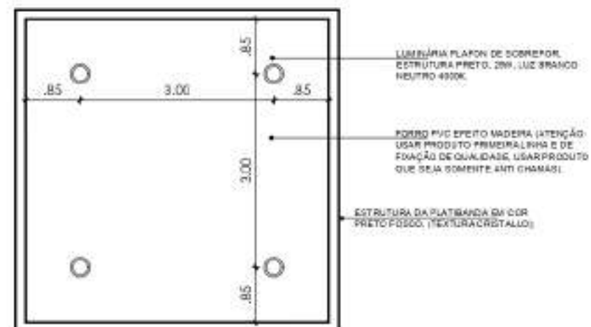
FORRO + LUMINOTÉCNICO
