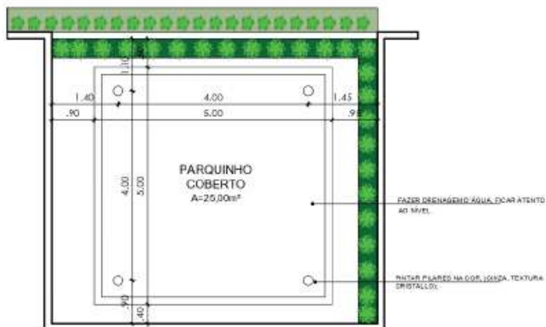
PLANTA BAIXA
